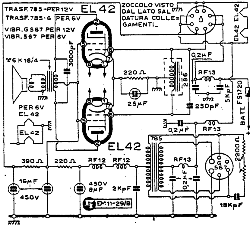
GALLO ING. G. - Autoradio Mod. S 5/AR Parte alimentazione
