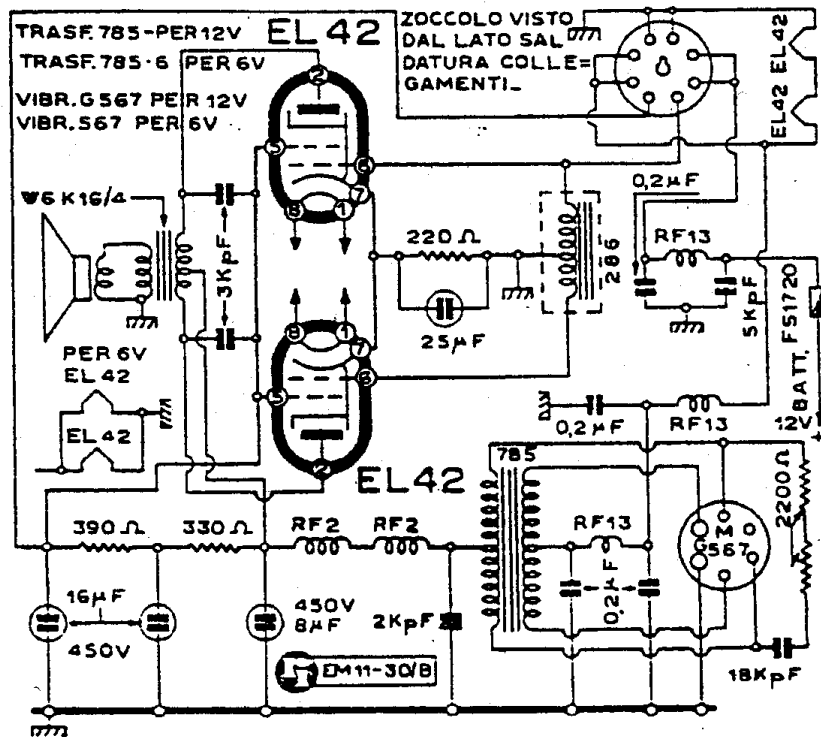
GALLO ING. G. - Autoradio Mod. S 5/AS Parte alimentazione
